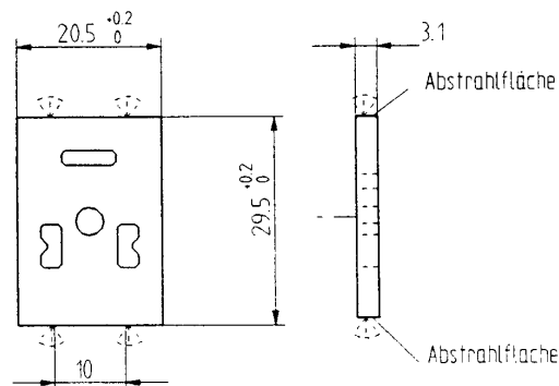
Bauform B
