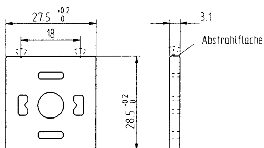
Bauform A
