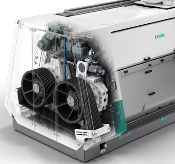
Seitenansicht des Overdrive-Systems mit dem neu entwickelten Riemenwechselmechanismus.
