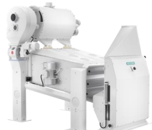
Separador e pré-limpador à ar recirculante com canal de aspiração
