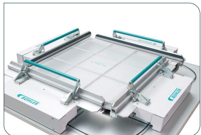
Siebspannvorrichtung NOVATENS.
