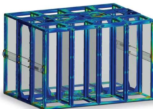
FEM-Berechnungen des Arenit Sichterrahmens.
