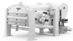
装有循环风选器的 重力分级去石机
